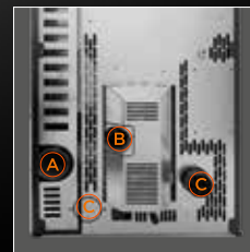
A Sortie Fumées B Entrée air de combustion C Sortie de canalisation
