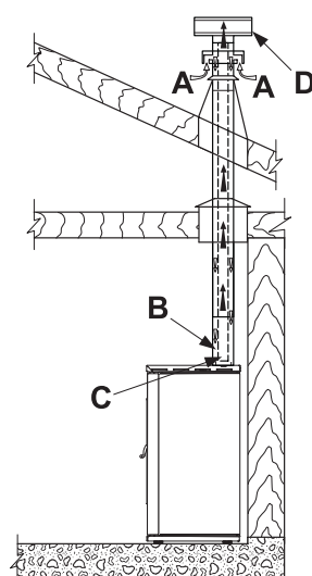
fig. 5.5 INSTALLAZIONE USCITA FUMI SUPERIORE
