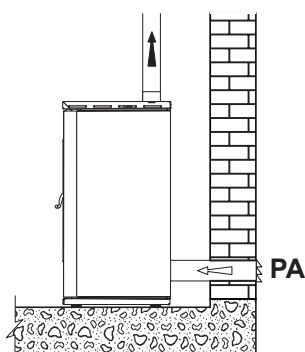
fig. 5.6 INSTALLAZIONE USCITA FUMI SUPERIORE
