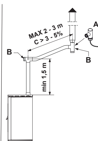
fig. 5.7 INSTALLAZIONE USCITA FUMI SUPERIORE
