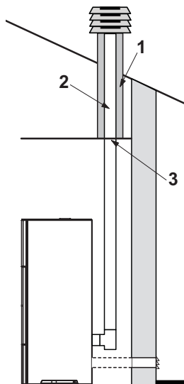
fig. 5.9 INSTALLAZIONE USCITA FUMI SUPERIORE
