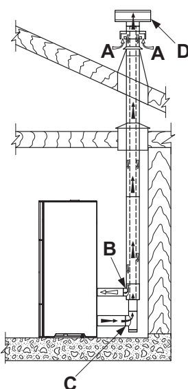
fig. 5.5 INSTALLAZIONE USCITA FUMI POSTERIORE
