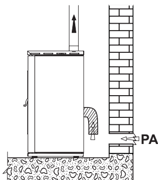
fig. 5.3 INSTALLAZIONE USCITA FUMI SUPERIORE
