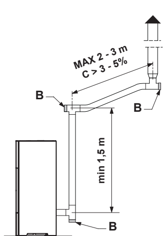
fig. 5.7 INSTALLAZIONE USCITA FUMI POSTERIORE
