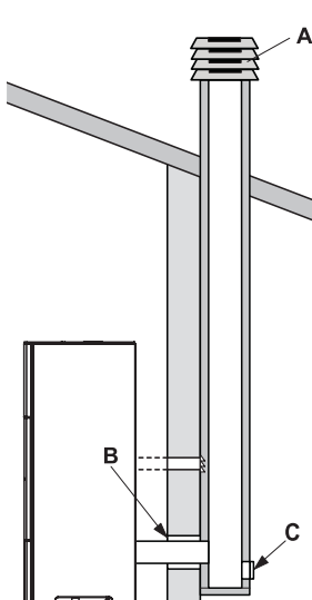
fig. 5.8 INSTALLAZIONE USCITA FUMI SUPERIORE
