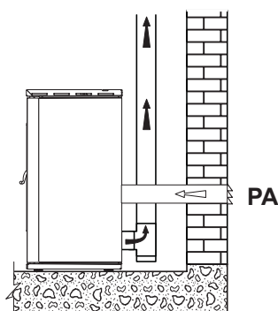
fig. 5.6 INSTALLAZIONE USCITA FUMI POSTERIORE
