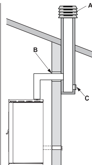
fig. 5.8 INSTALLAZIONE USCITA FUMI POSTERIORE
