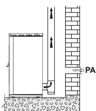
fig. 5.3 INSTALLAZIONE USCITA FUMI POSTERIORE
