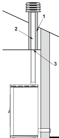
fig. 5.9 INSTALLAZIONE USCITA FUMI POSTERIORE
