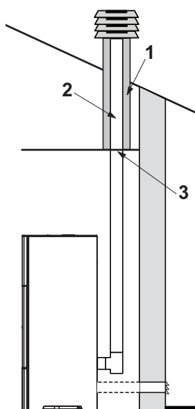
fig. 5.9 INSTALLAZIONE USCITA FUMI SUPERIORE
