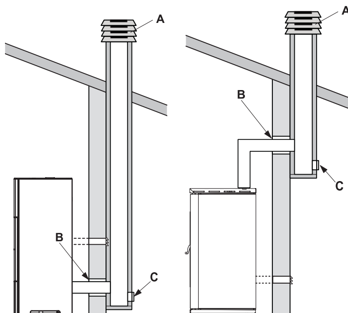
fig. 5.8 INSTALLAZIONE USCITA FUMI SUPERIORE
