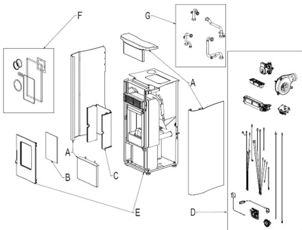
Dessin éclaté
