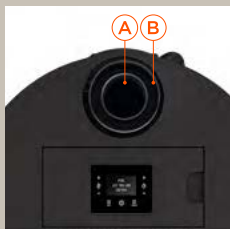
Sortie Coaxiale Poujoulat A Sortie des fumées B Entrée d'air comburant
