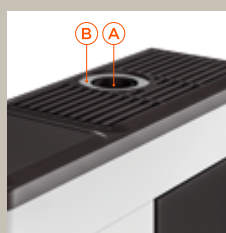
Scarico Coassiale Poujoulat A Uscita fumi B Entrata aria comburente
