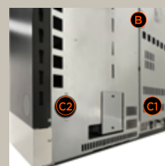
B Entrata aria comburente C1 - C2 Uscite Canalizzabili
